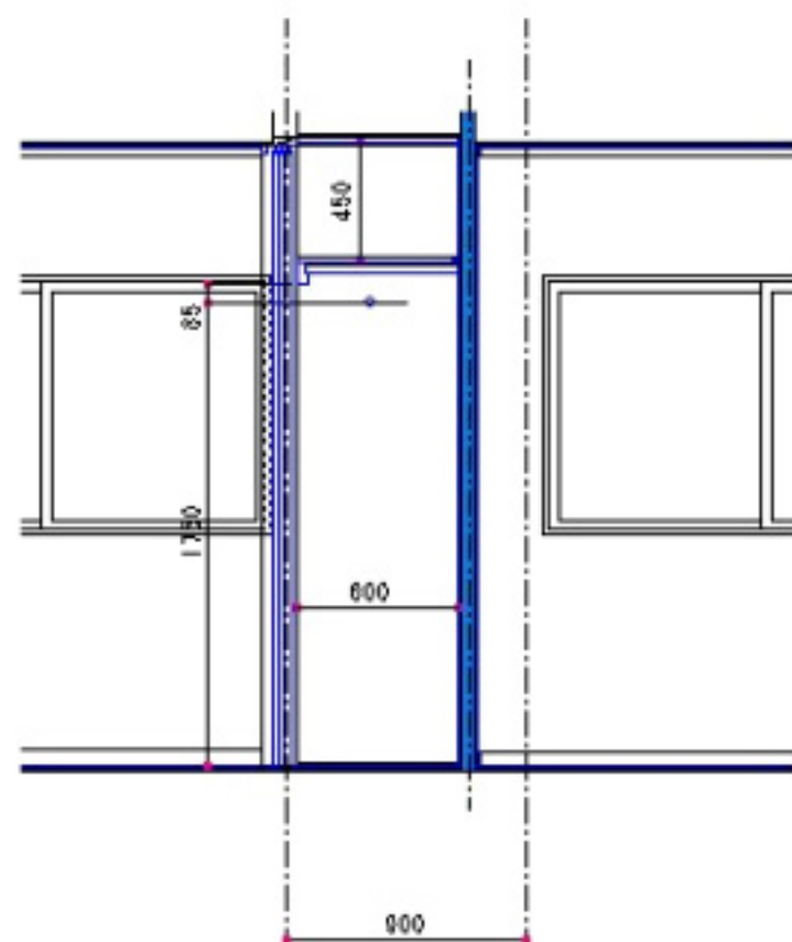
クロゼット断面図
